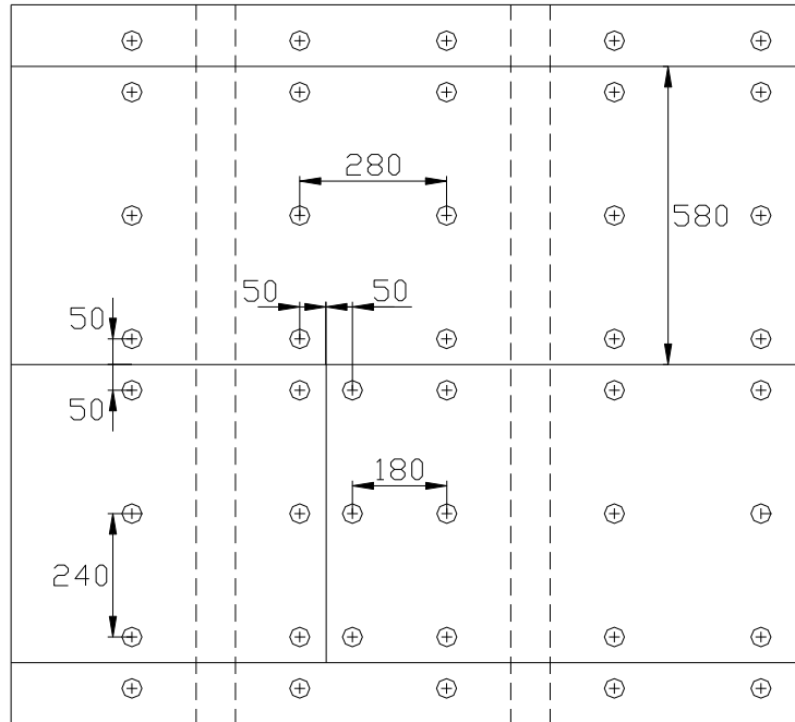
Section C-C 1/10 :
