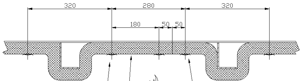
Section C-C 1/10 :
